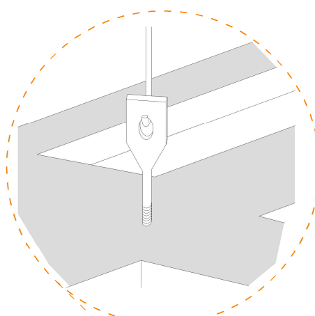
DETALLE 2 PUNTO DE ANCLAJE
